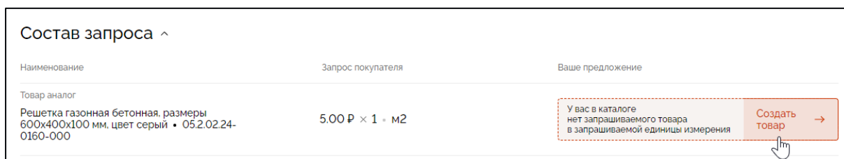
Рисунок 111 – Создание товара в вашем каталоге для предложения по запросу котировок
