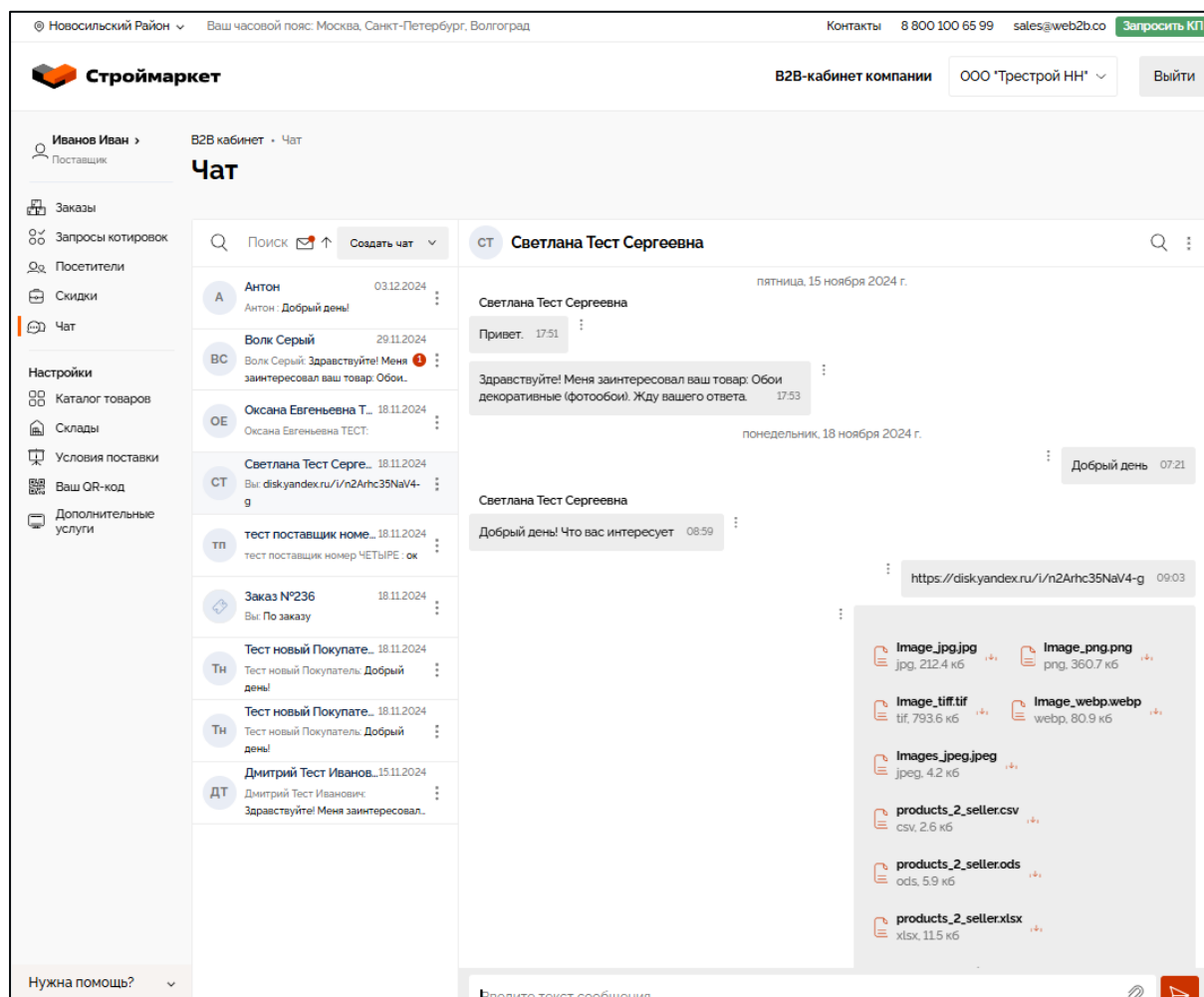
Рисунок 42 – Беседа в чате
